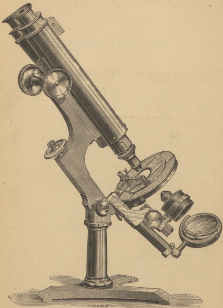
H. SEBALD ZENTMAYER'S NEW MODEL U. S. A. H. MICROSCOPE.
