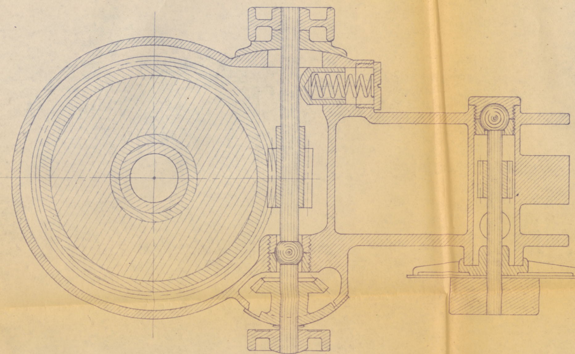
— Section F-F —
