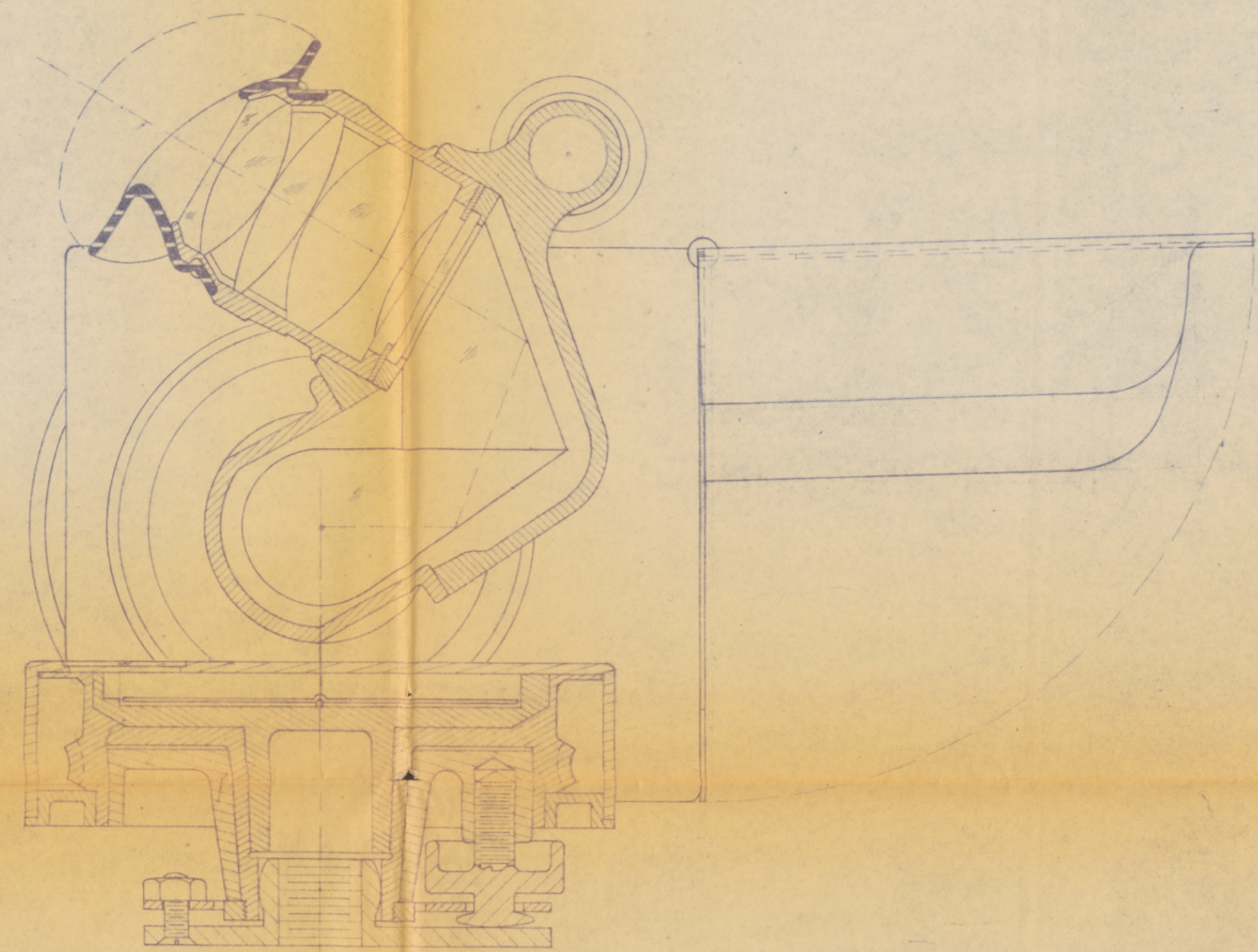
— Section A-A —
