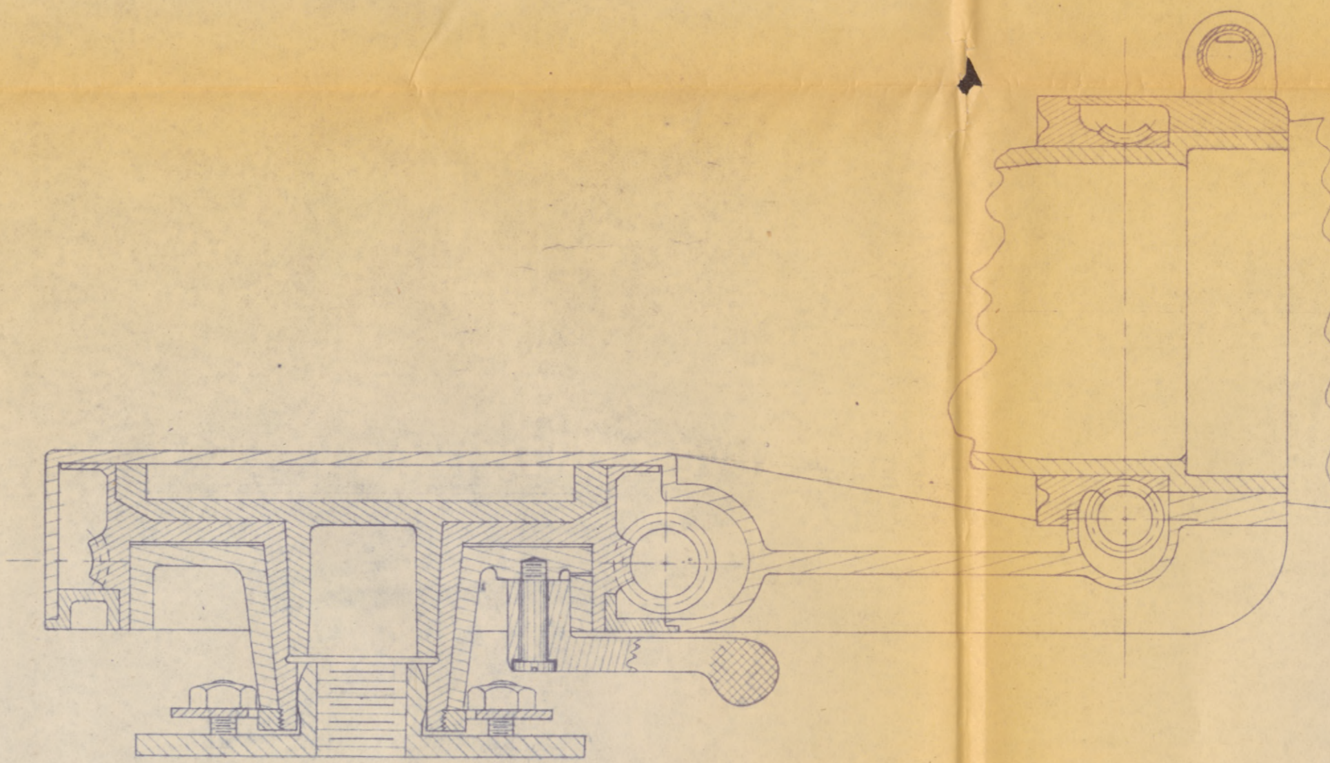
— Section E-E —
