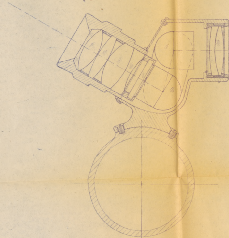
— Section B-B —
