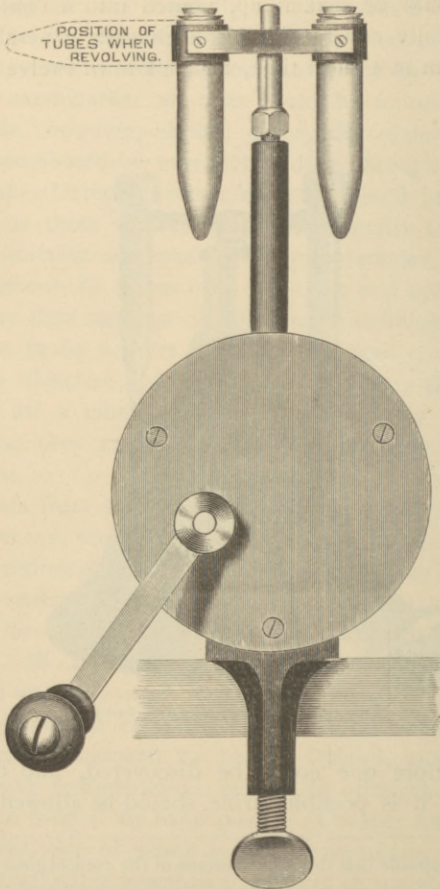
FIG. 45.—The Daland Centrifuge.
