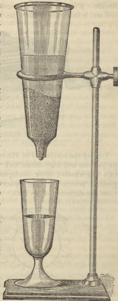
FIG. 3. DISPLACEMENT APPARATUS.
